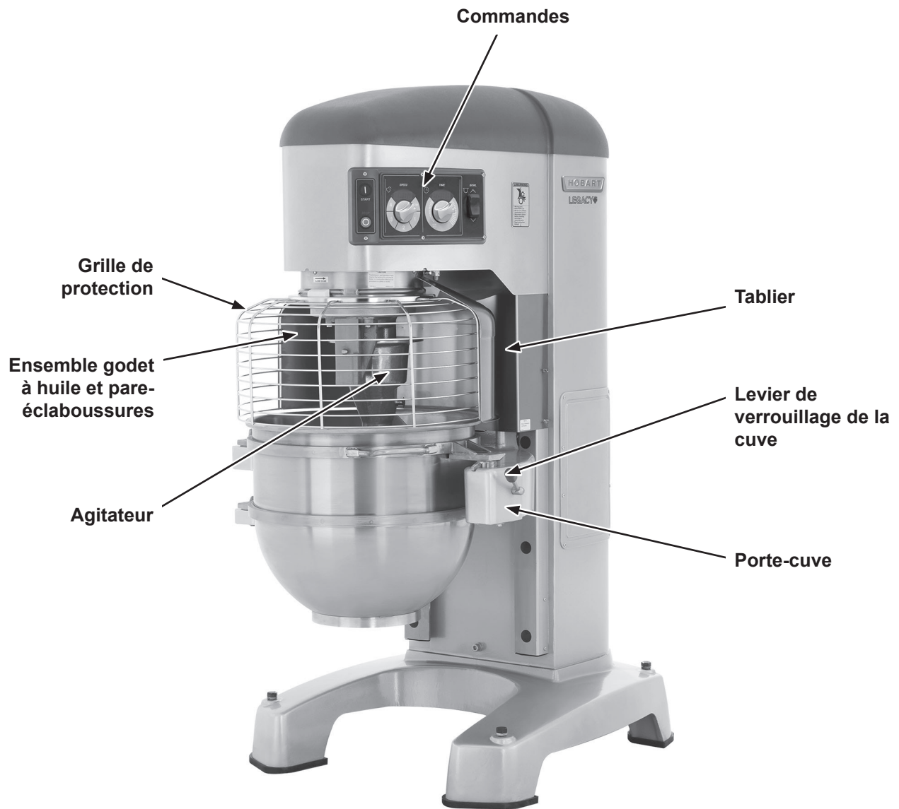
Batteur-mélangeur de 80 ptes
