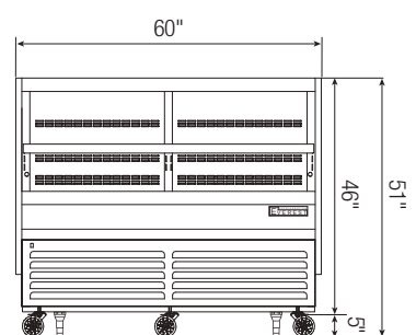
EOMH-60-W(B)-35-T
