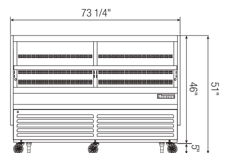
EOMH-72-W(B)-35-T
