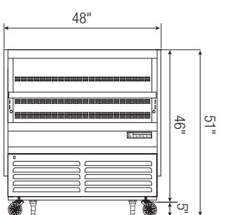
EOMH-48-W(B)-35-T
