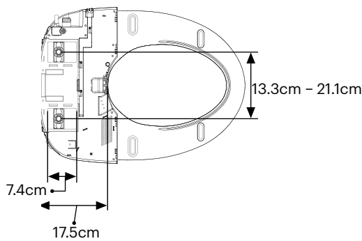
Vista inferior
