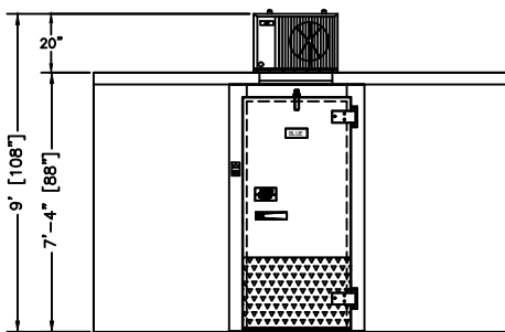
ELEVATION RIGHT HINGE
