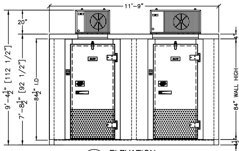
1 ELEVATION SCALE: 1/4"=1'-0"
