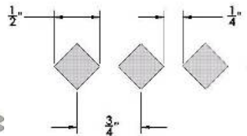
GRATE-DIA24
