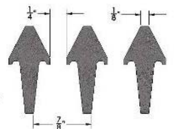
GRATE-CSTR24
