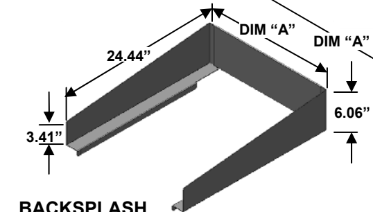
BACKSPLASH
