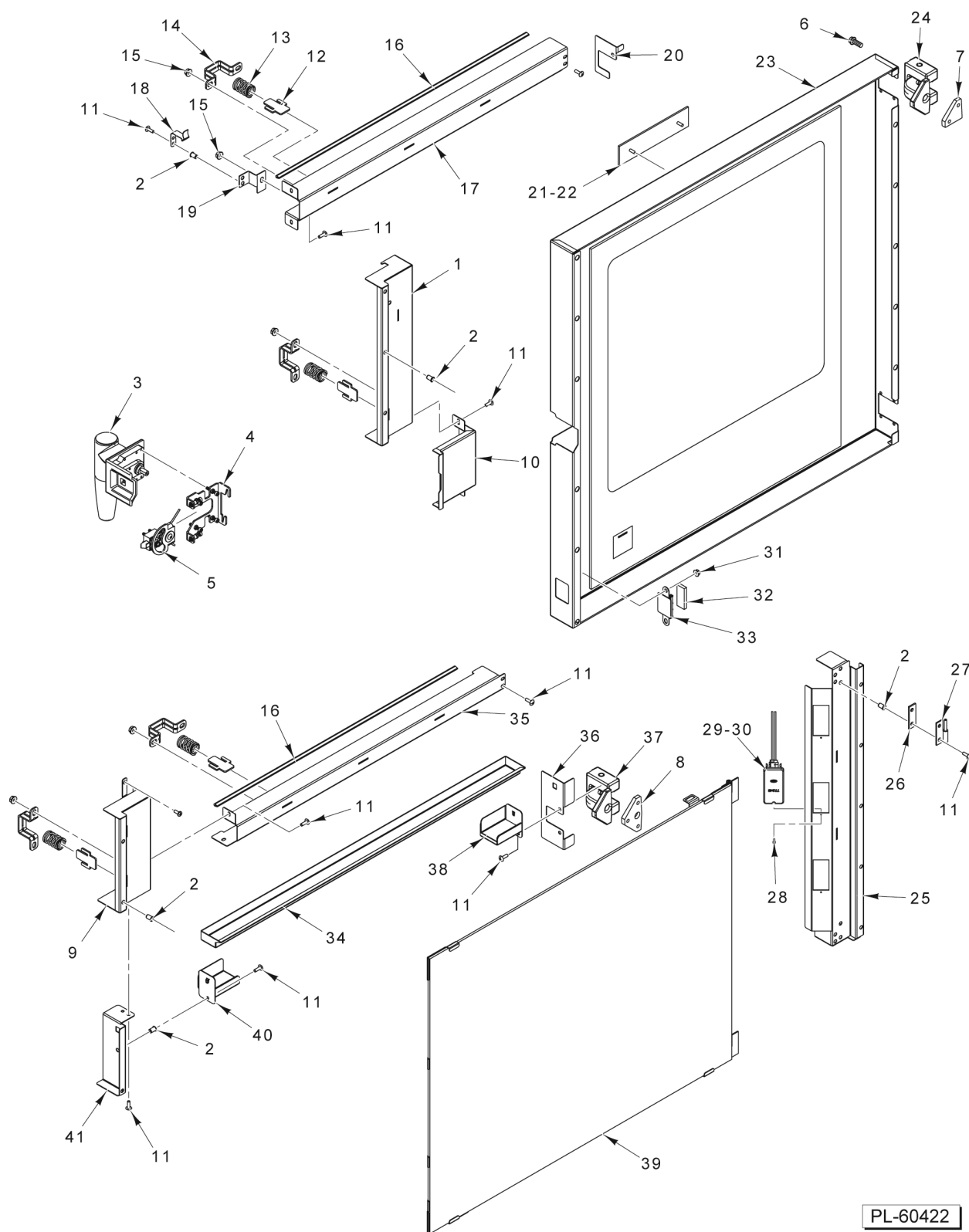
DOOR ASSEMBLY (BEFORE SN 541082623)
