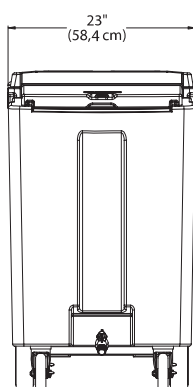
ICS200 Front/Width
