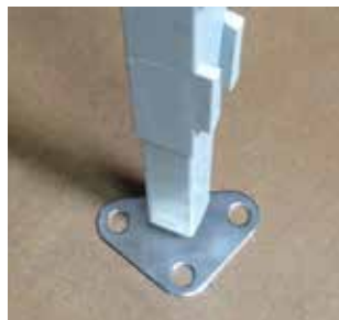
Seismic Foot
