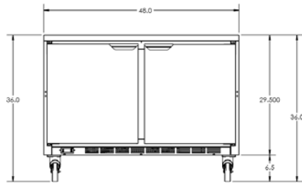
00C31-038A 6" CASTERS - STANDARD 401-249A / 401-250D 00A31-034D-03 LEVELER
