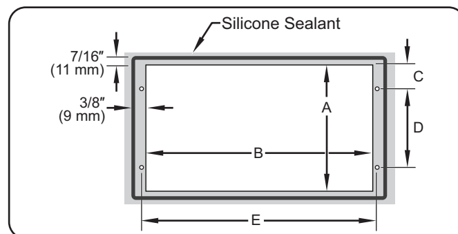
Dimensions de la découpe de la série RMB2
