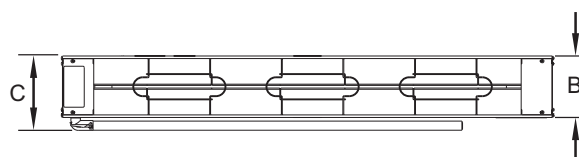
Vue de dessous — Modèle GRAM
