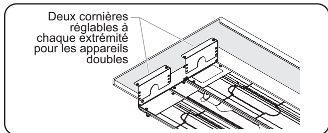
Montage des unités doubles
