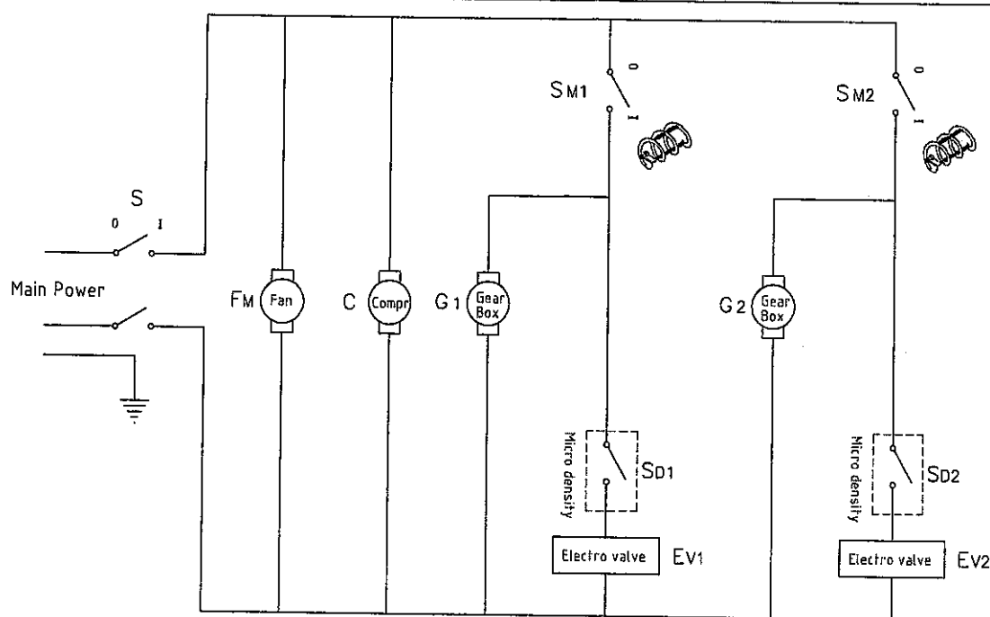
OASIS 2-10 Schema Elettrico - Schemas - Esquemas - Schéma - Elektrik "BASIC"
