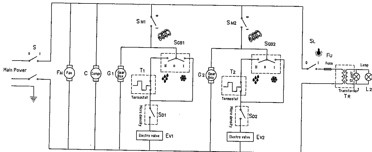
OASIS 2-10 Schema Elettrico - Schemas - Esquemas - Schéma - Elektrik "STANDARD"
