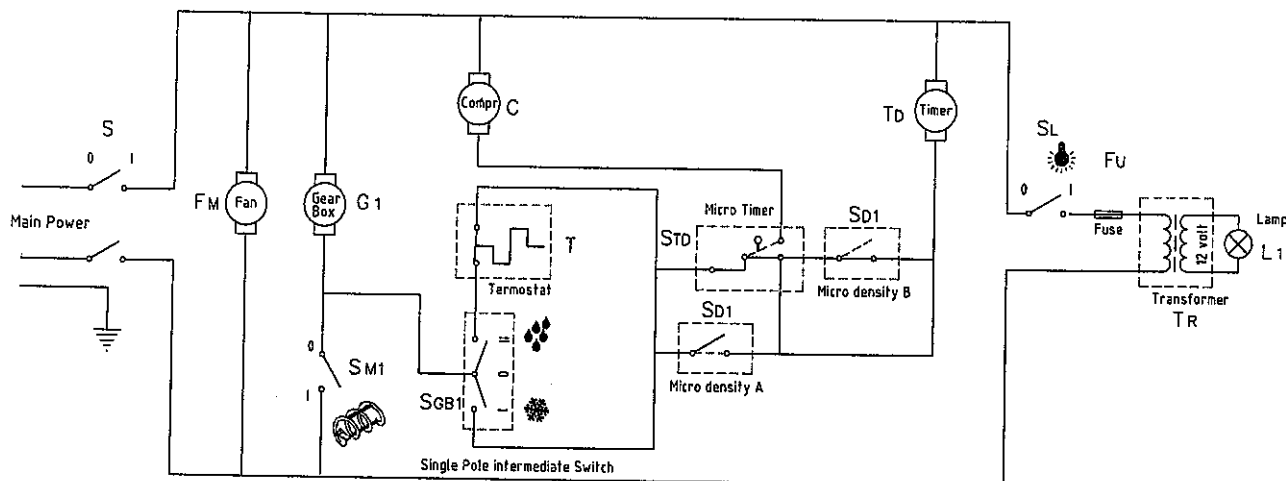
OASIS 1-10 Schema Elettrico - Schemas - Esquemas - Schéma - Elektrik "STANDARD"
